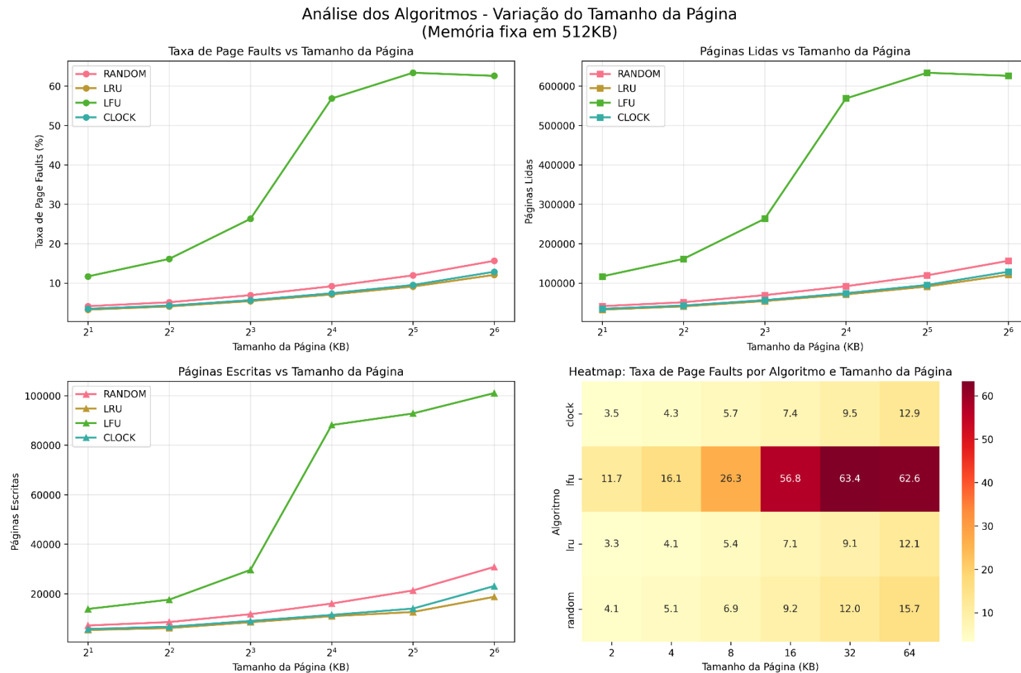
Figura 2 – Análise dos Algoritmos: Variação do Tamanho da Página (Memória fixa em 512KB)
