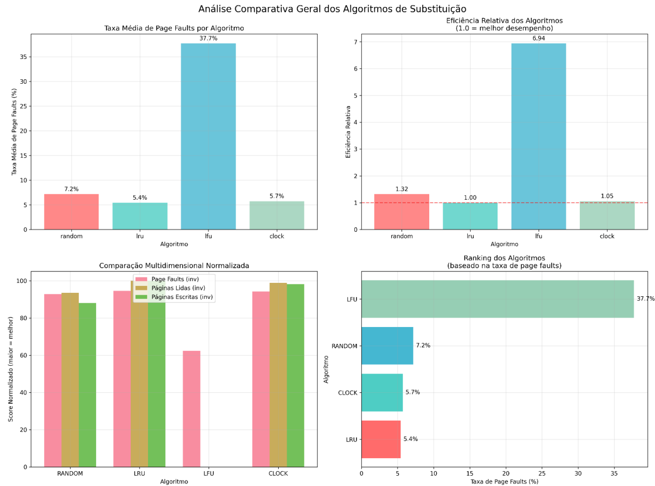
Figura 4 – Análise Comparativa Geral dos Algoritmos de Substituição
