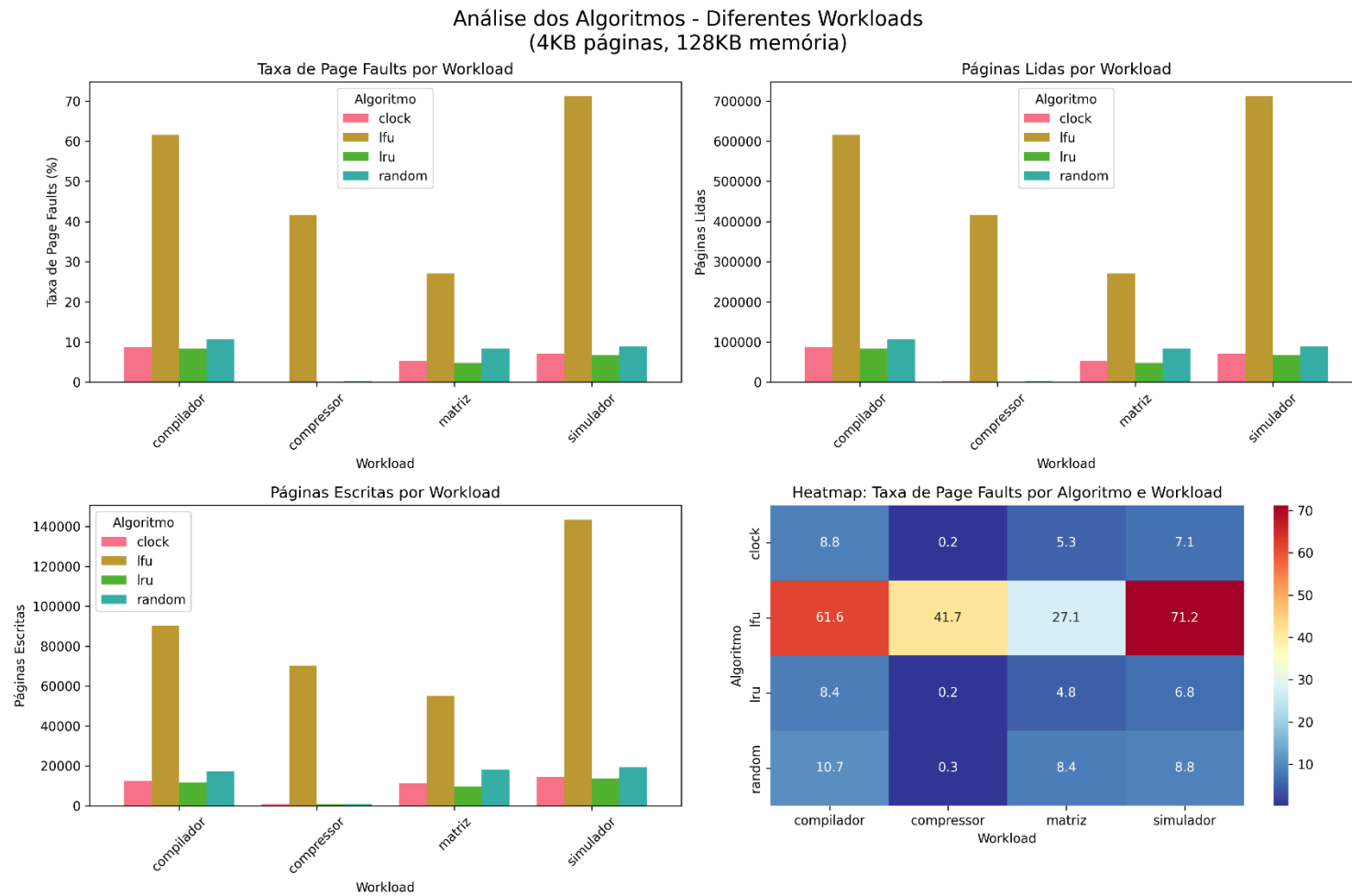
Figura 3 – Análise dos Algoritmos: Diferentes Workloads (4KB páginas, 128KB memória)
