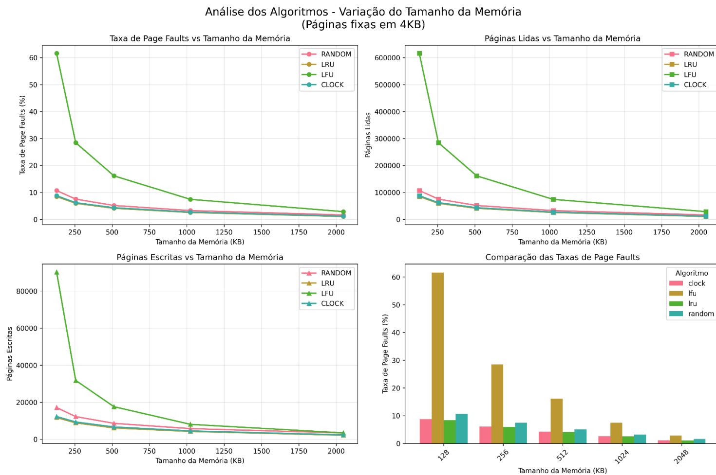
Figura 1 – Análise dos Algoritmos: Variação do Tamanho da Memória (Páginas fixas em 4KB)
